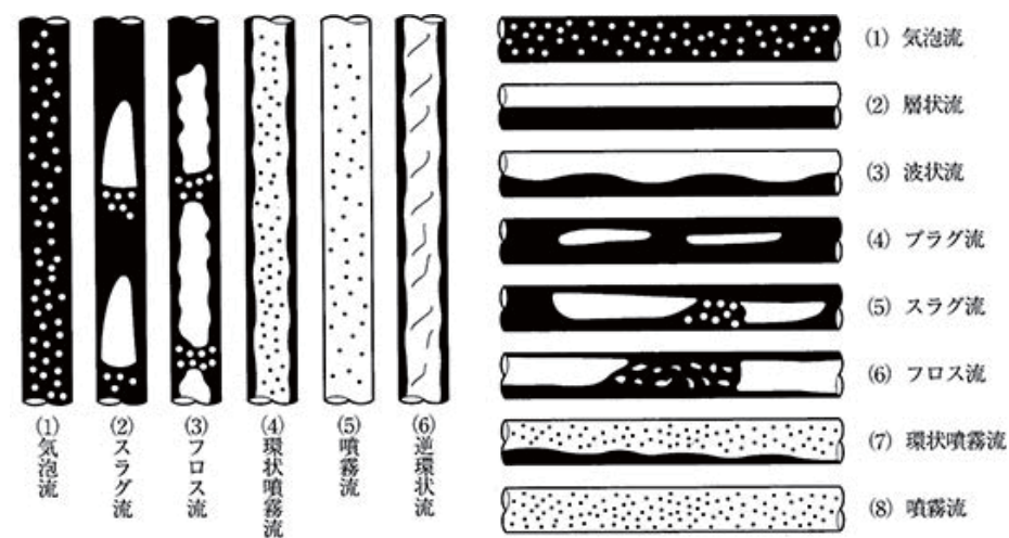
図 4.1-11 垂直管中の流動様式
